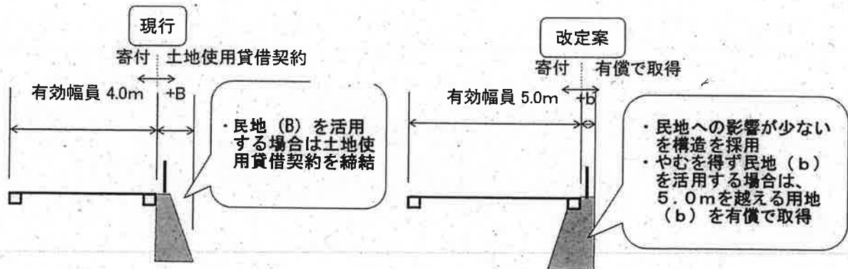
図-2 下法面擁壁の構造と用地
