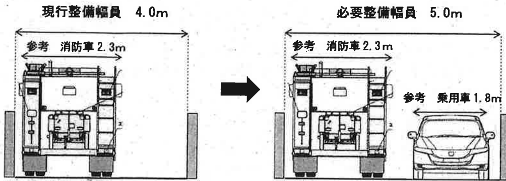
図-1 必要幅員
