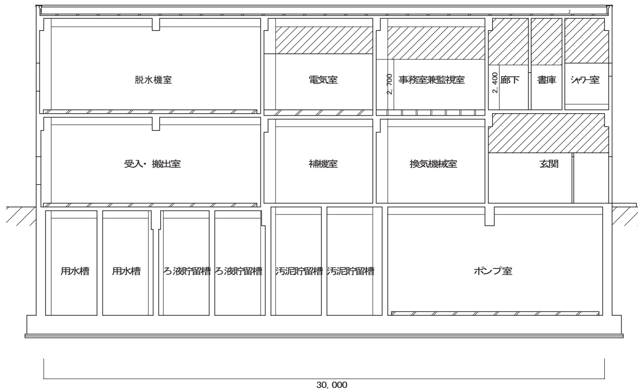
東西 断面図
