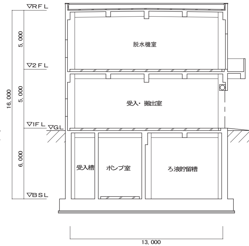
南北 断面図
