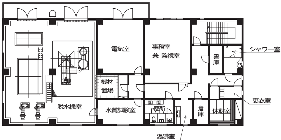
2階平面図
