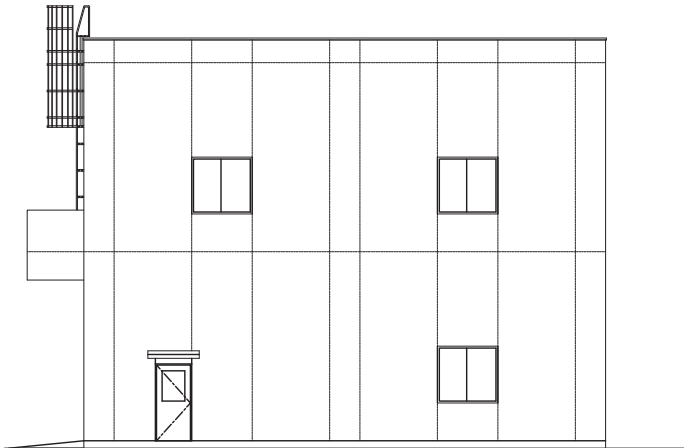
東側立面図
