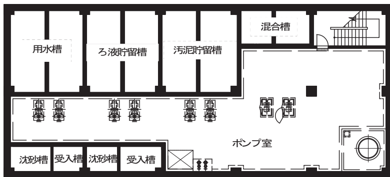
地下1階平面図
