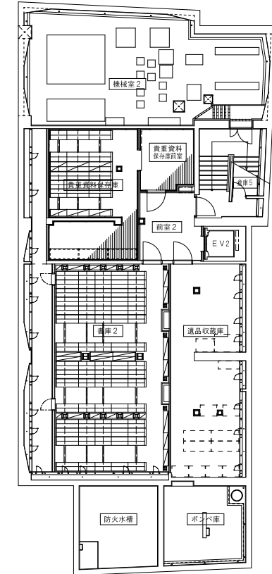
地下2階平面図
