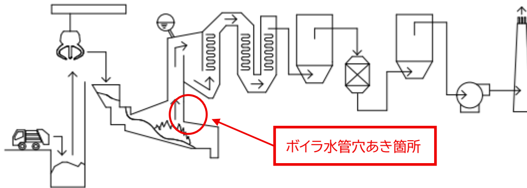
【図1】焼却炉全体図
