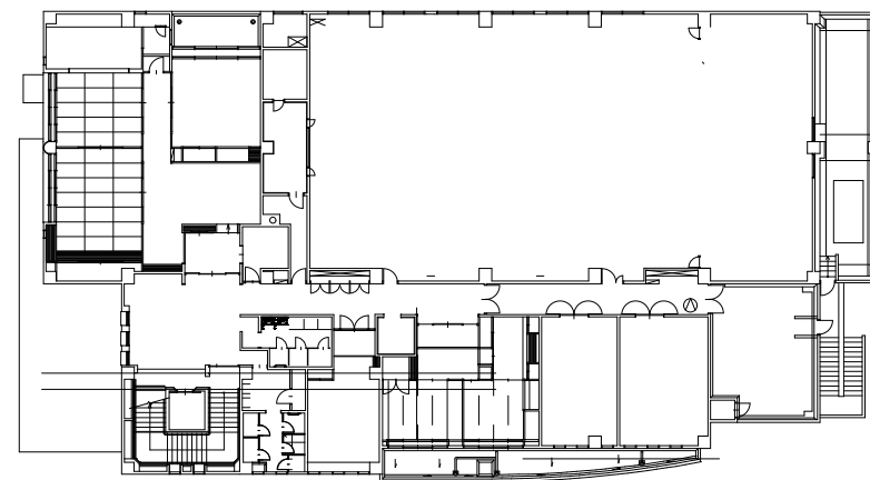
2階平面図
