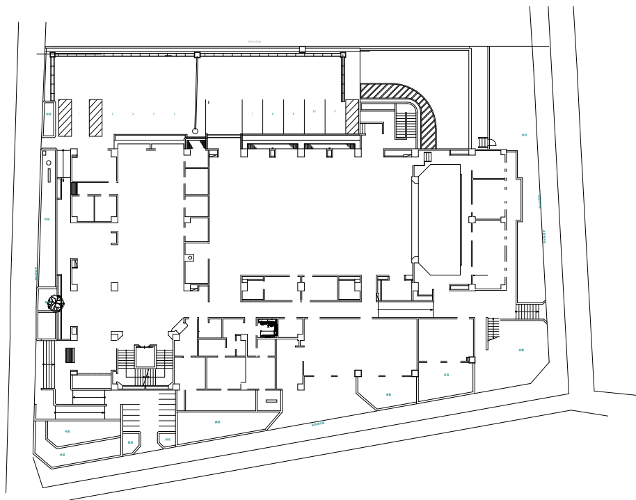
1階平面図
