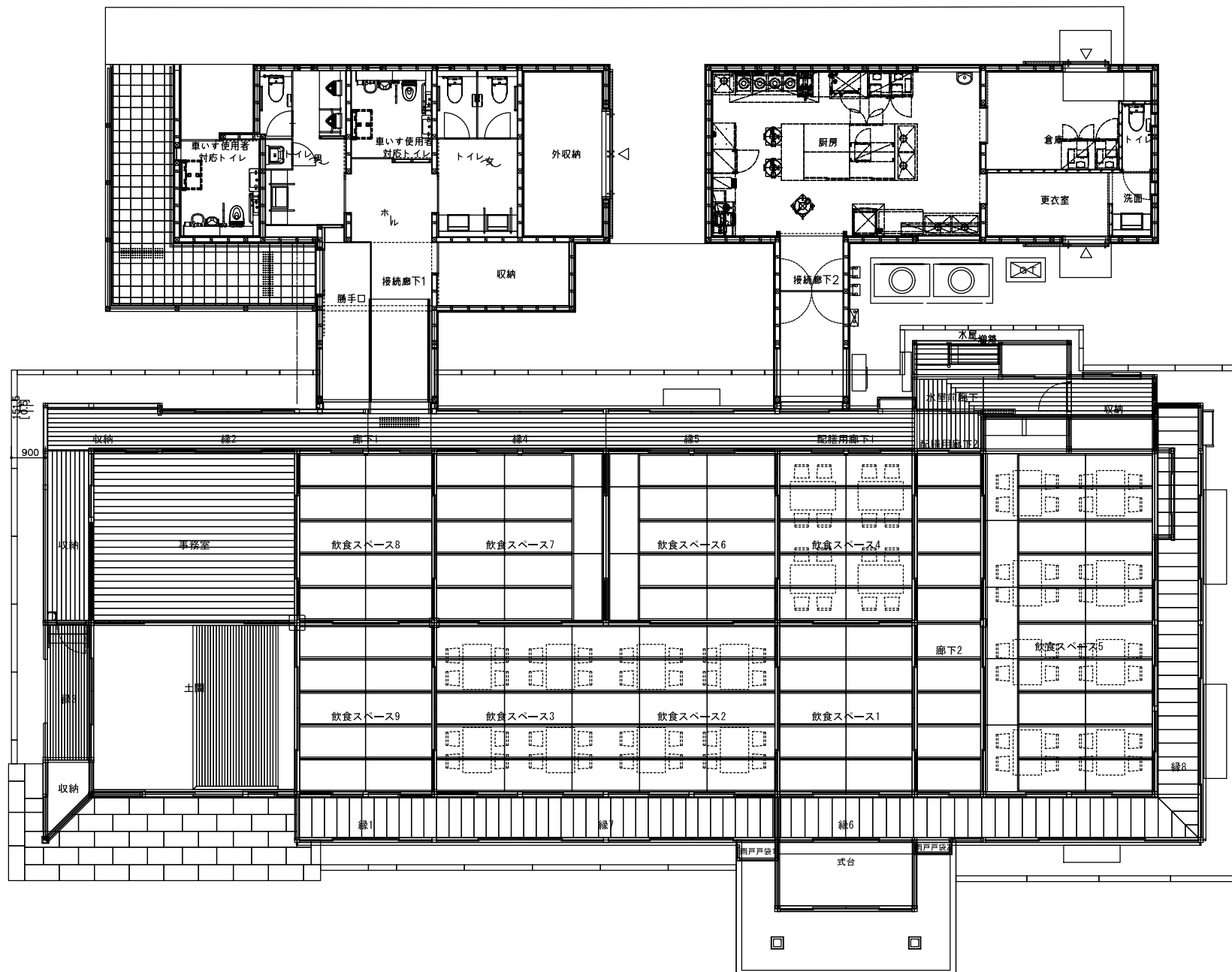
建築平面図
