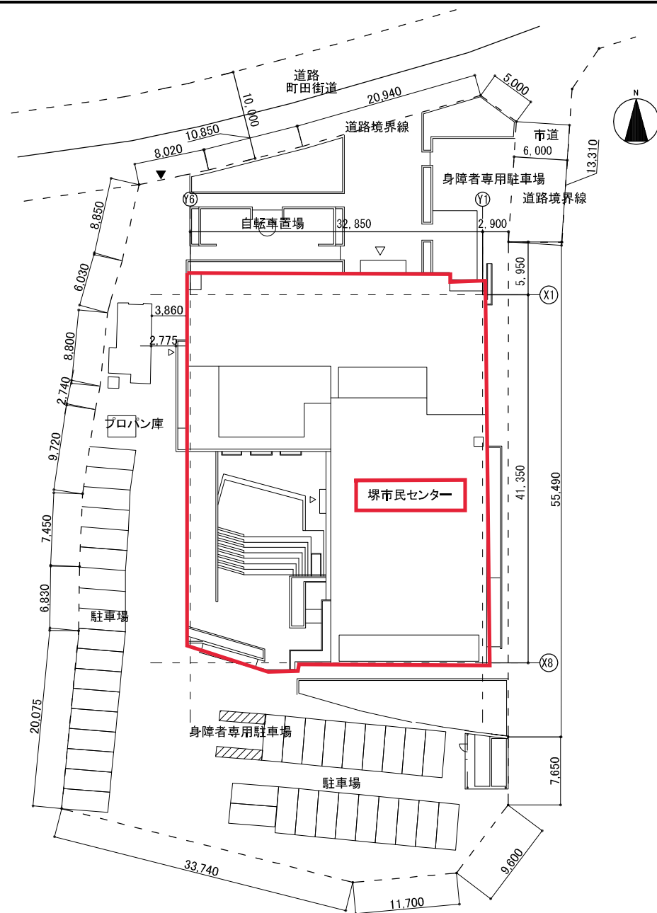
配置図 1:200
