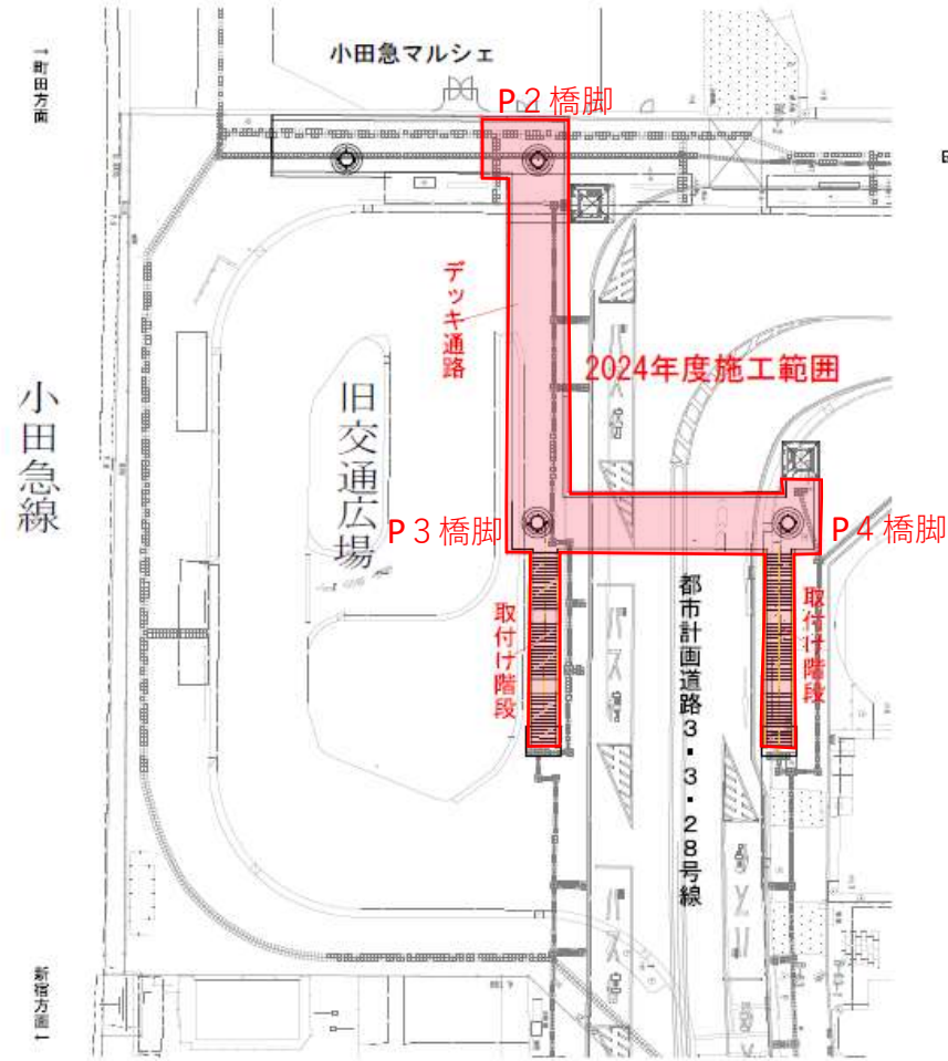
平面図
