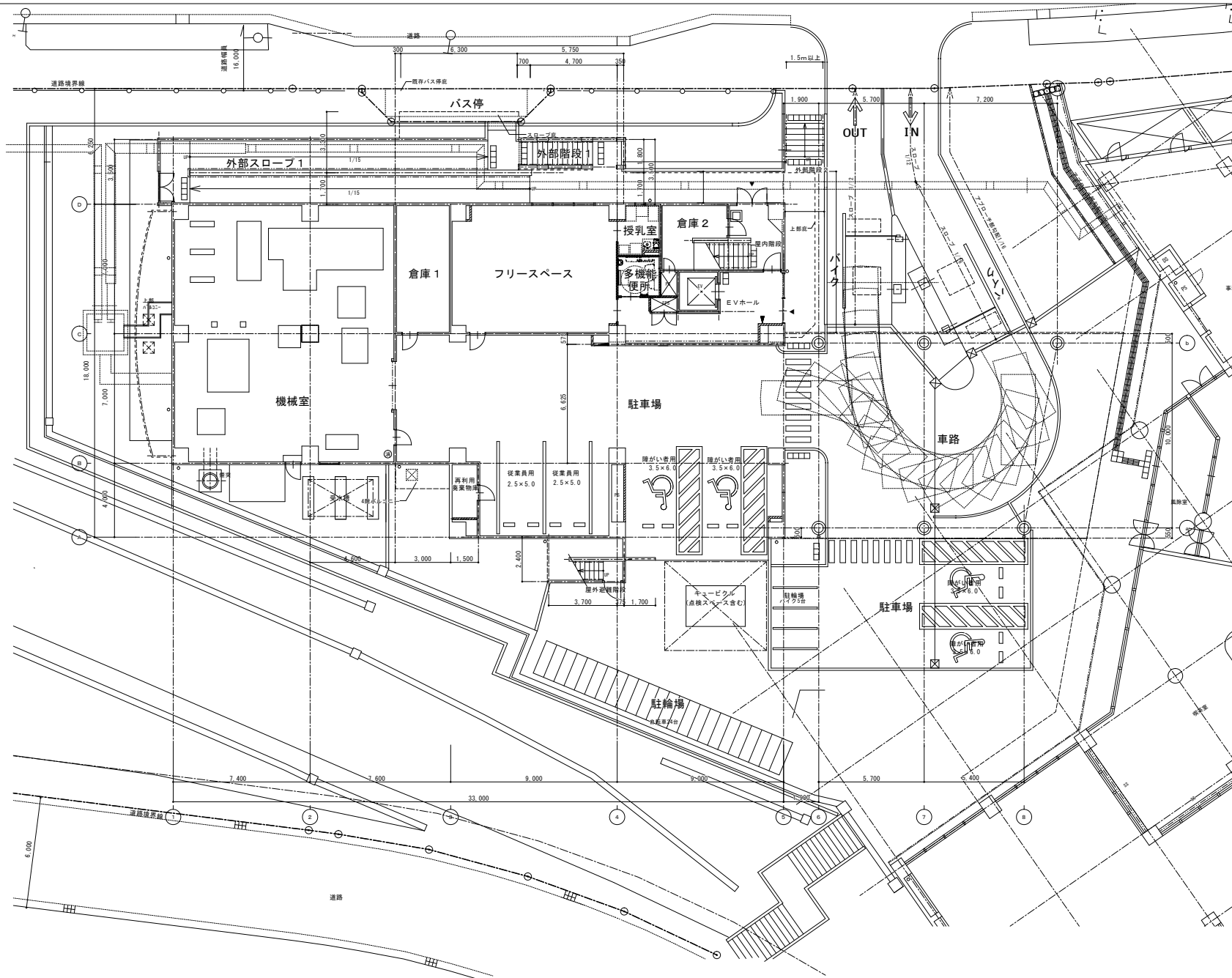
1階平面図
