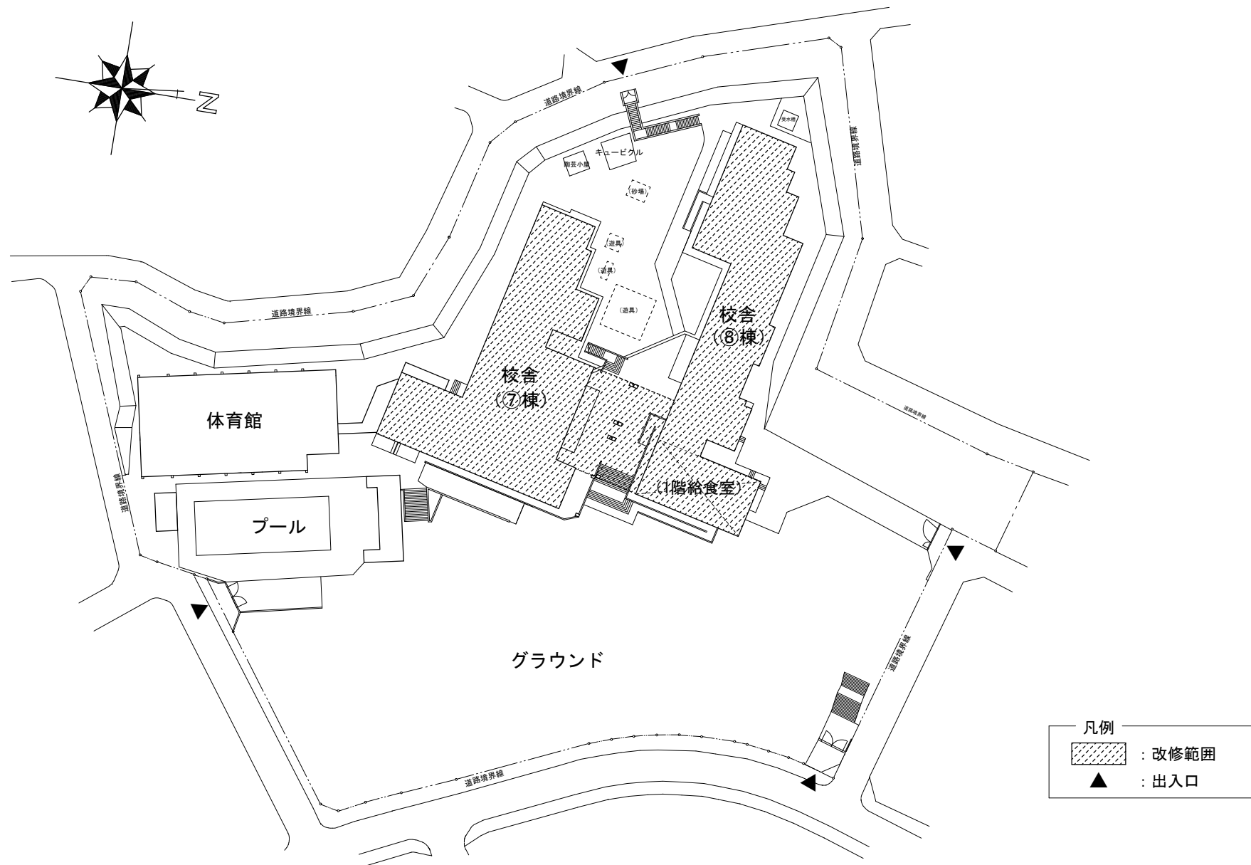
配置図
