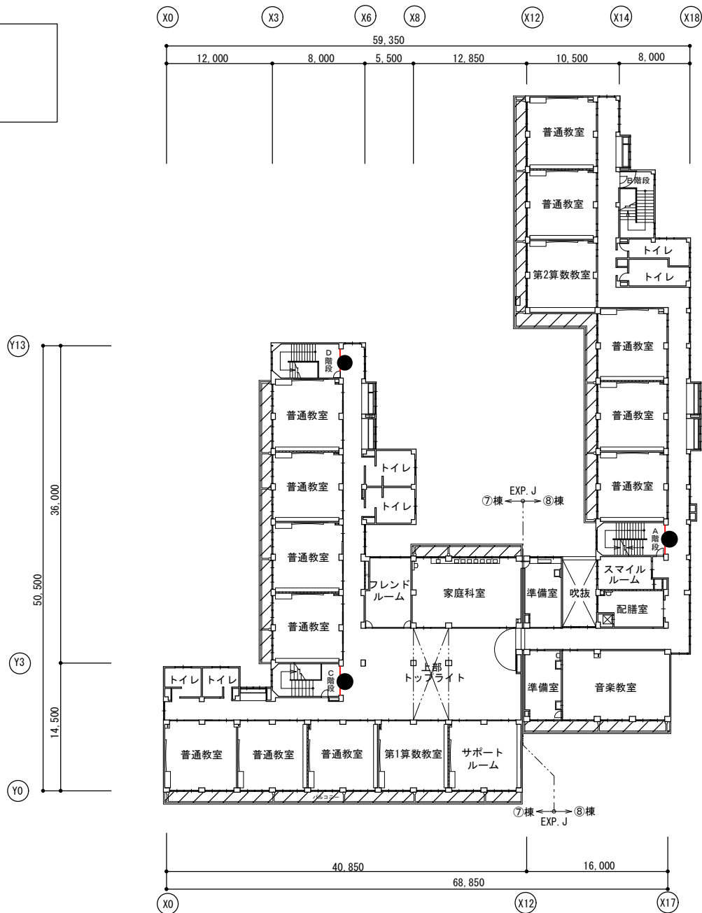
3 階 平 面 図
