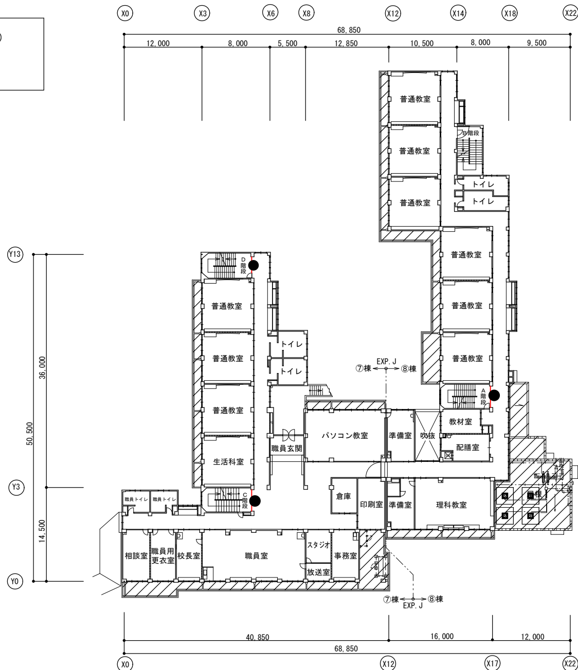
2 階 平 面 図
