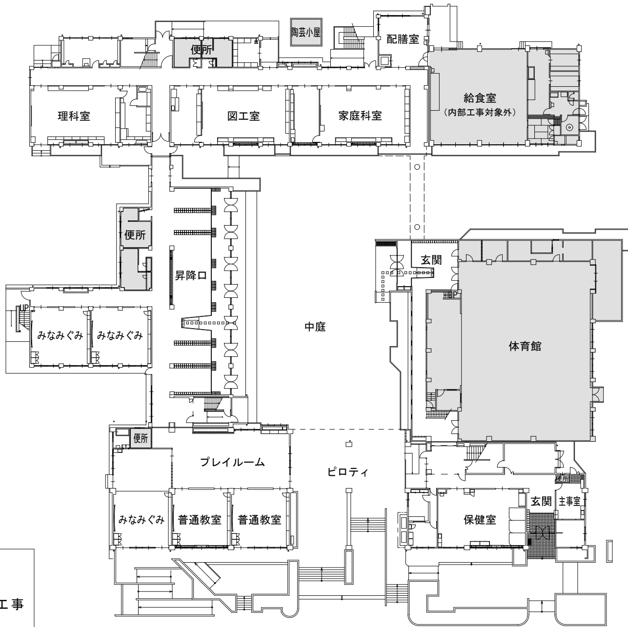
1階平面図
