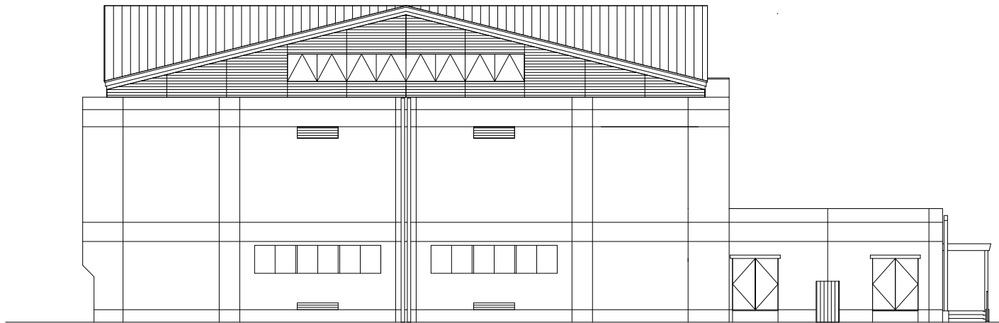
北側立面圖
