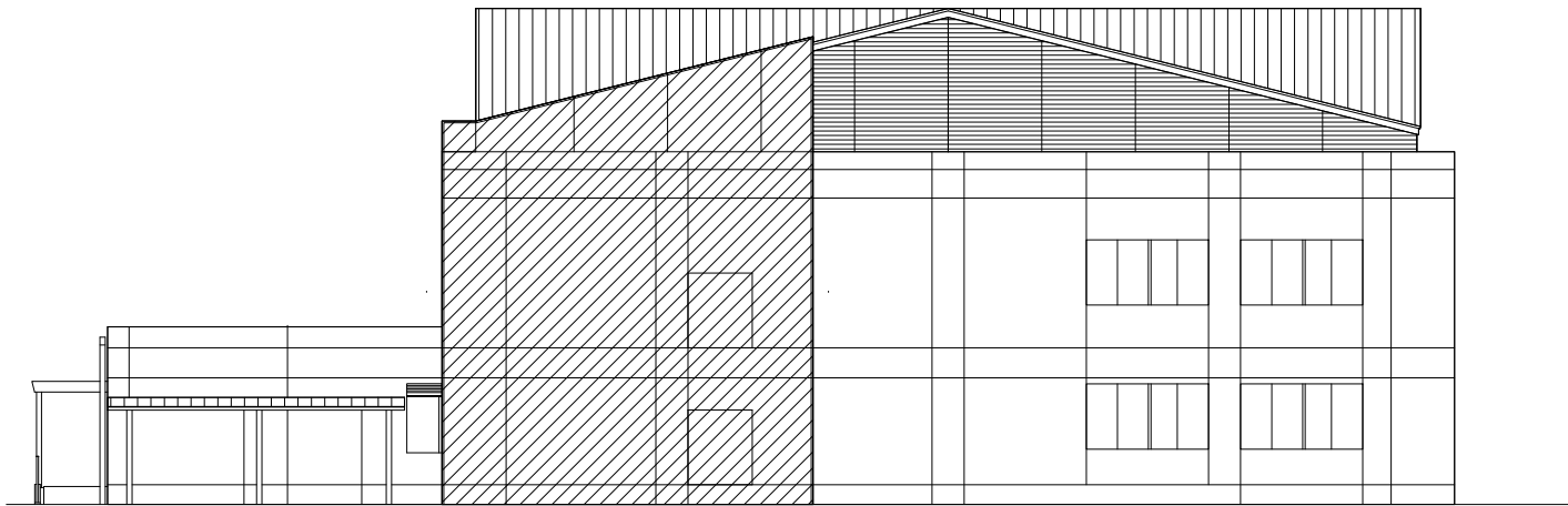
南側立面圖
