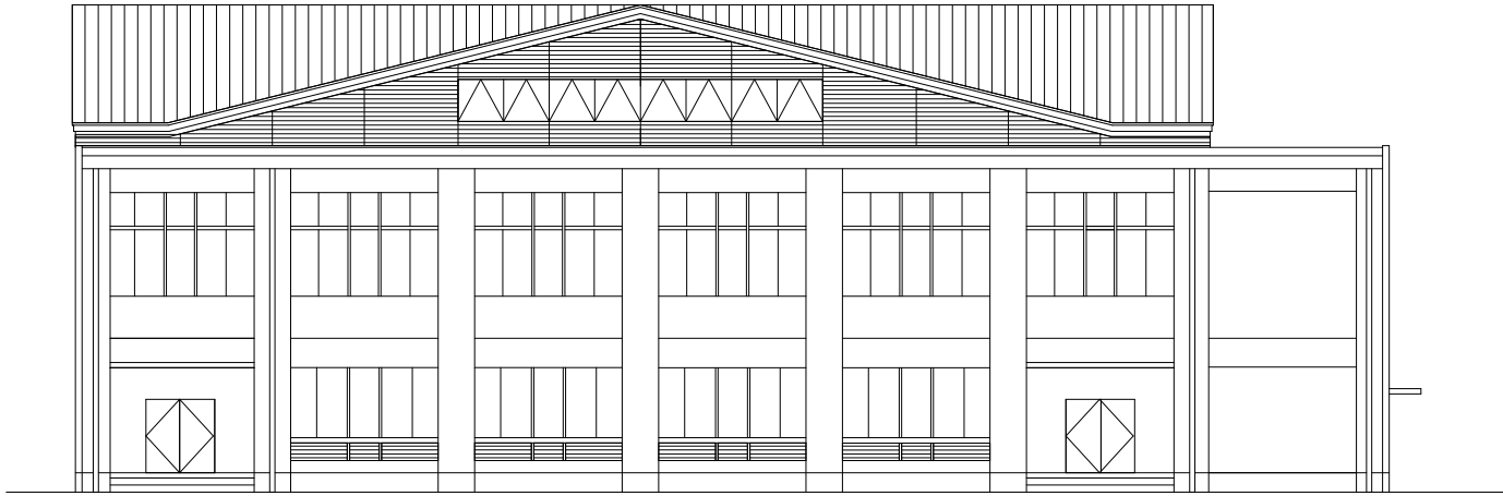
東側立面圖
