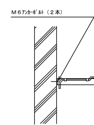
壁付けの場合
