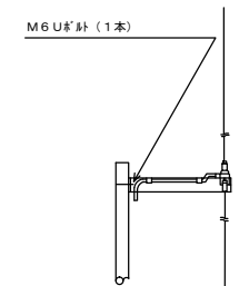
穴取付けの場合
