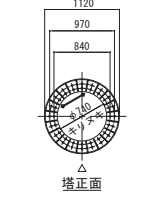
JOINT2 平面図
