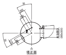
下部マンホール平面図
