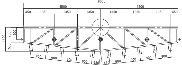
Z3 平面図
