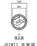
JOINT3 平面図
