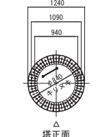
JOINT1 平面図
