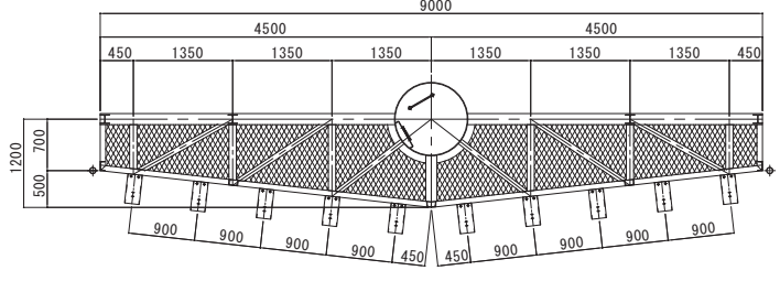
Z1 平面図
