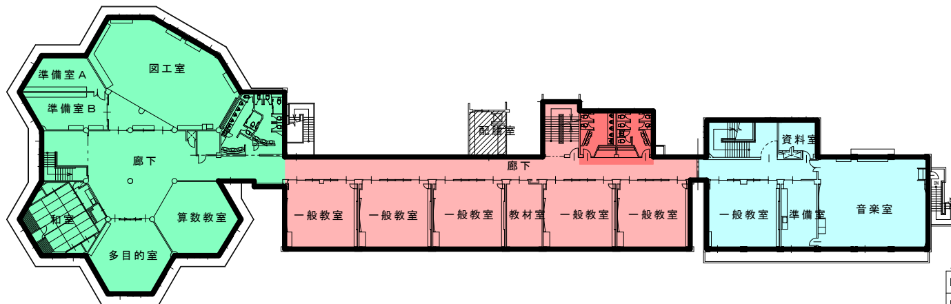
3階平面図
