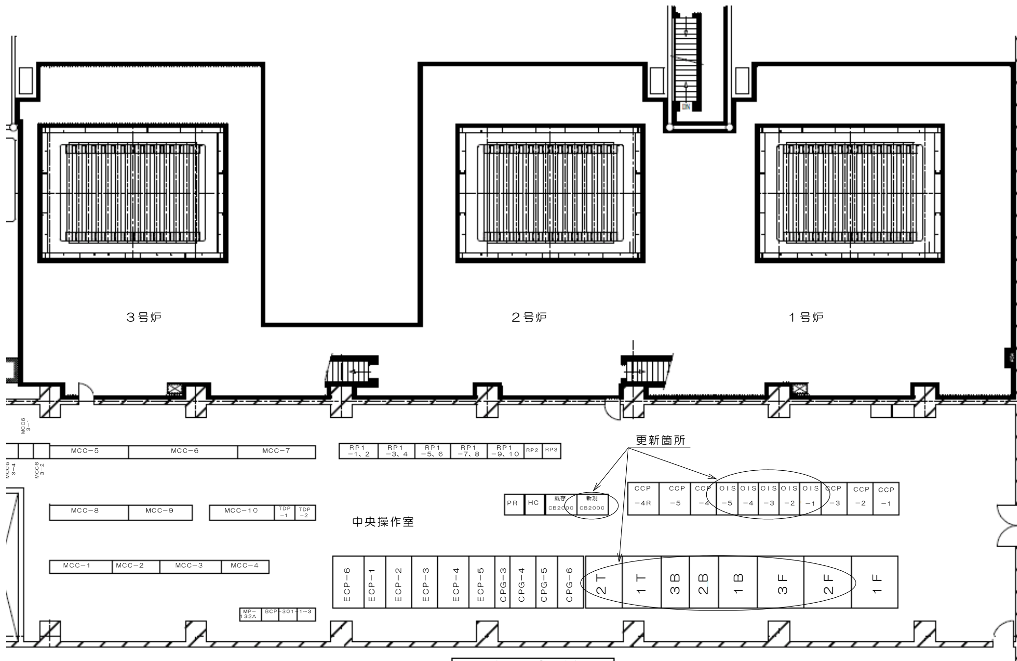
中央操作室詳細図
